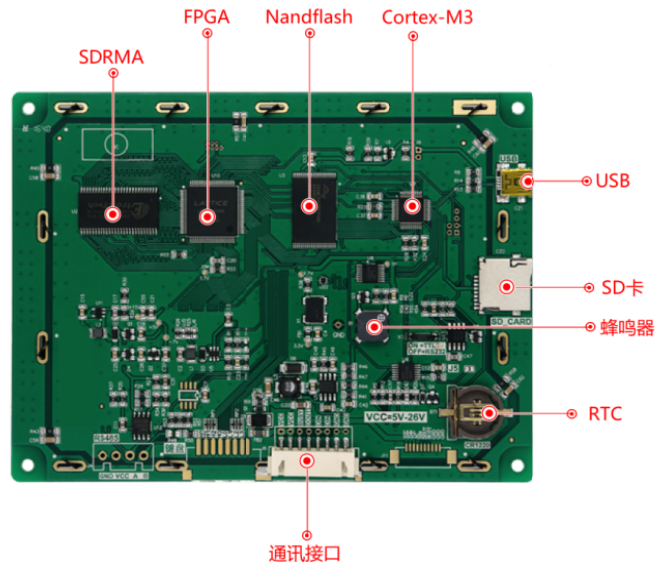
图 1-3 硬件配置图
