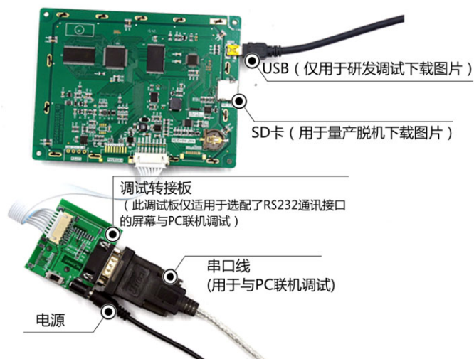
图 1-4 调试工具图
